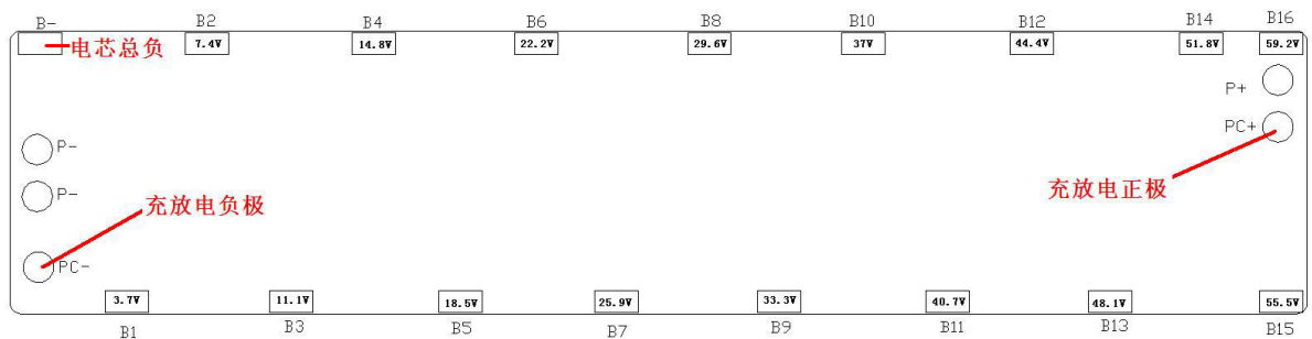
16串同口接线图
