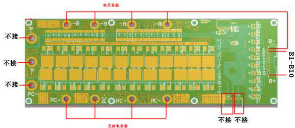
10串同口接线图
