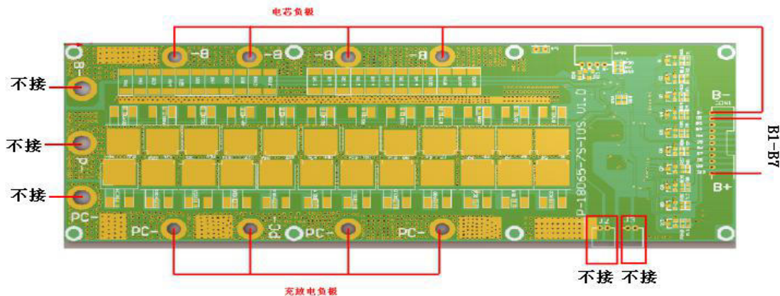
7串同口接线图
