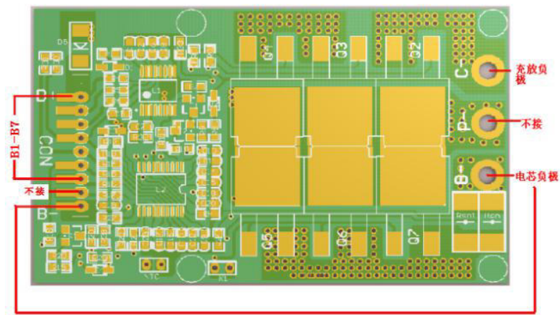
7串同口接线图
