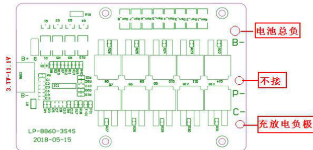
3串接线图
